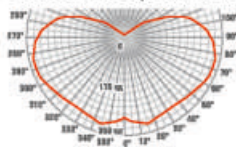
Тип КСС — Ш Класс светораспределения — П
