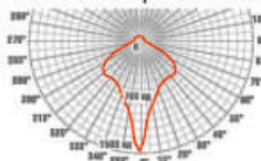
Тип КСС — Г Класс светораспределения — П
