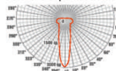
Тип КСС — К Класс светораспределения — П
