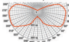
Тип КСС — Ш Класс светораспределения — Н
